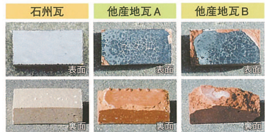
殆ど塩害が見られない石州瓦の試験体 塩害で素地の周辺がボロボロになった他産地の瓦 塩害で素地の半分がボロボロになった他産地の瓦
