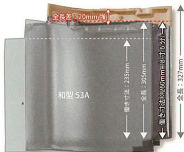
(53A との寸法比較図)
